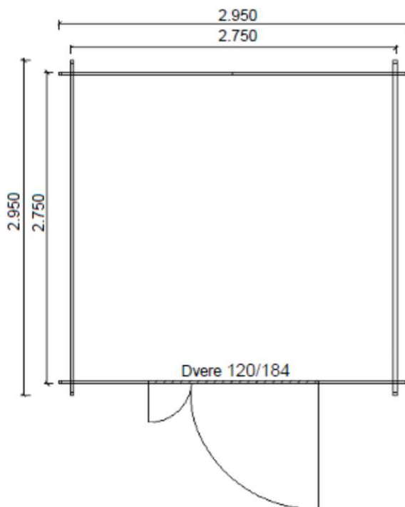
Pôdorys chatky:
