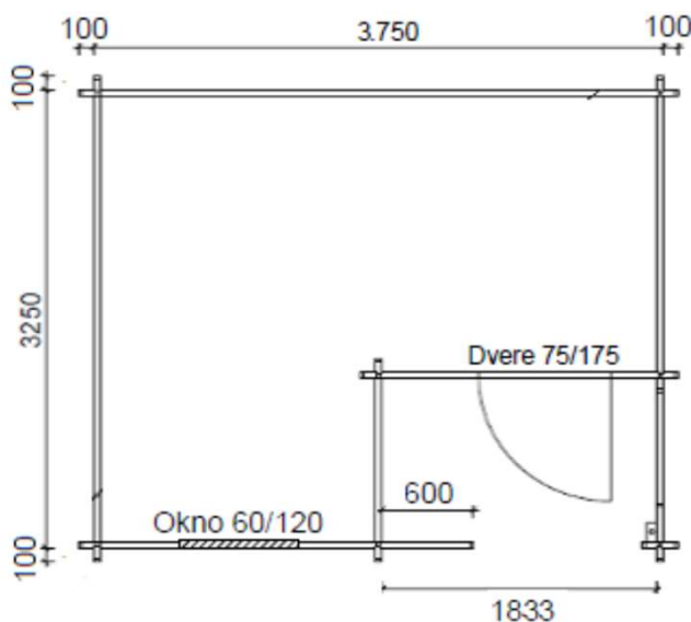
Pôdorys chatky:
