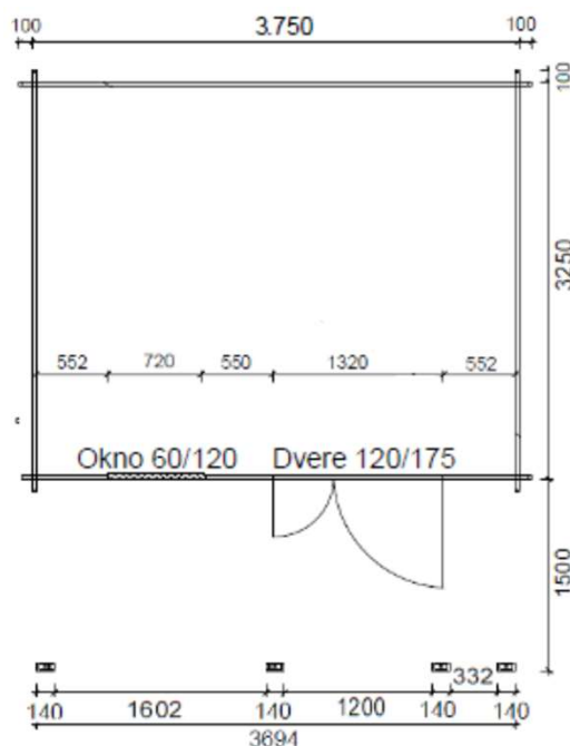
Pôdorys chatky:
