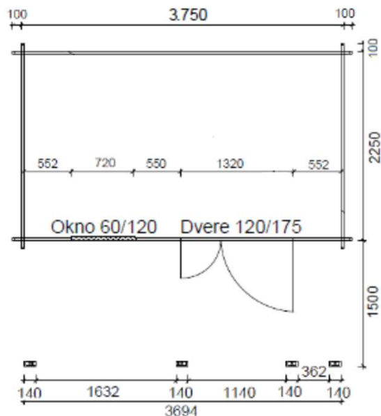
Pôdorys chatky:
