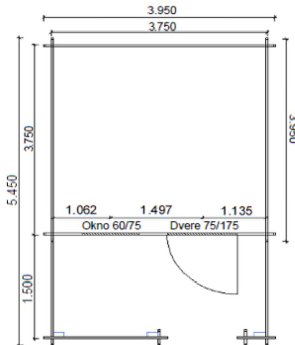
Pôdorys chatky:
