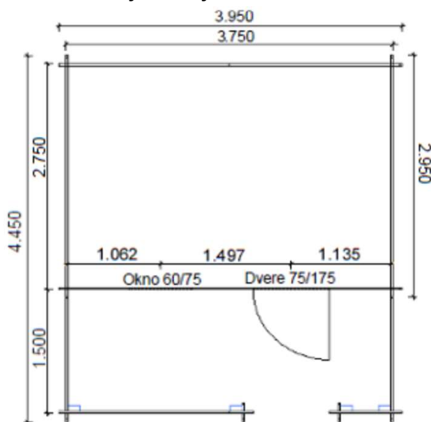
Pôdorys chatky:
