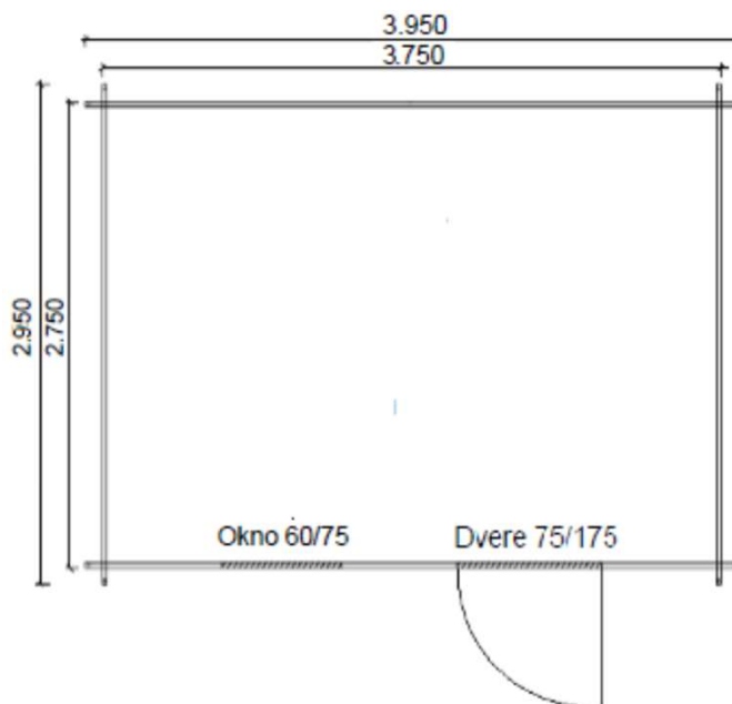
Pôdorys chatky:
