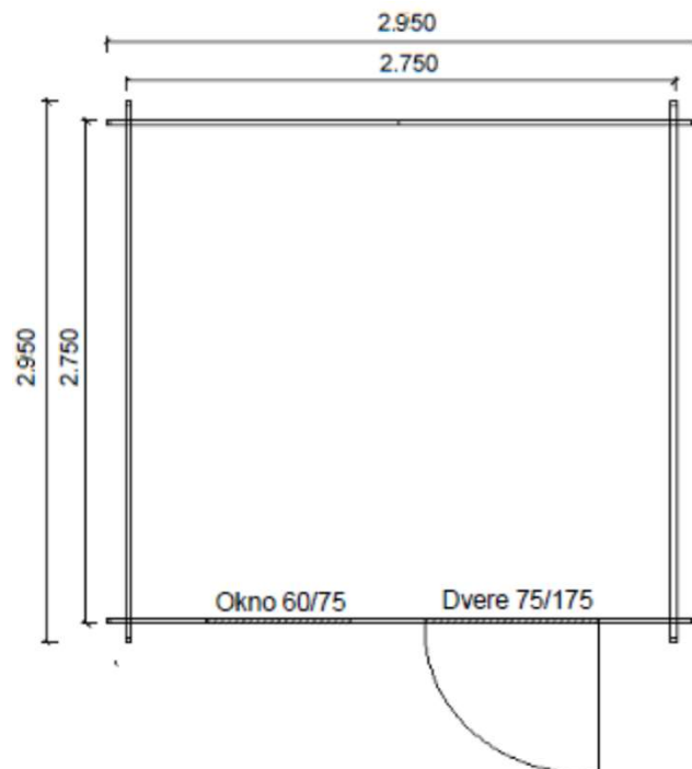
Pôdorys chatky:
