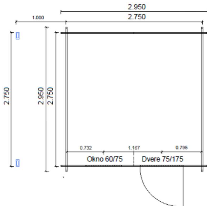
Pôdorys chatky:
