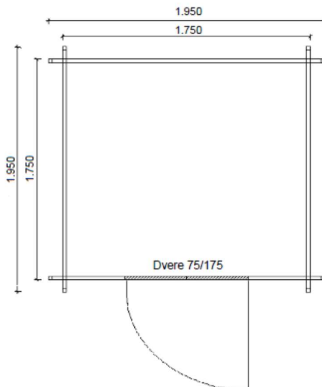
Pôdorys chatky:
