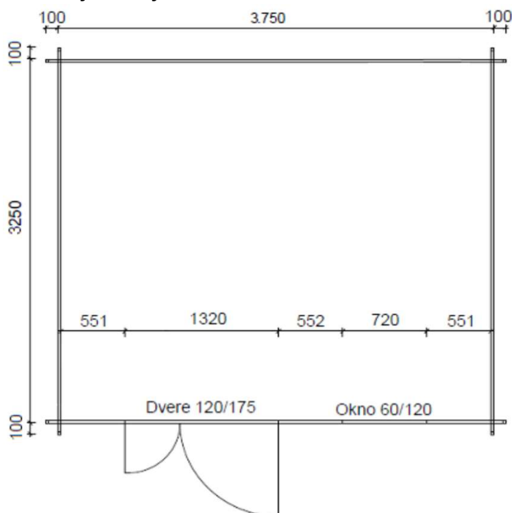
Pôdorys chatky:
