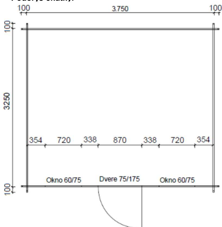
Pôdorys chatky:
